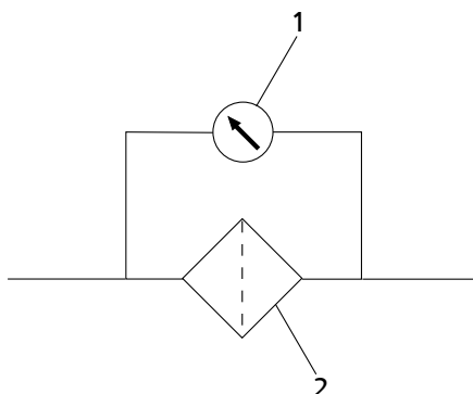
III. 5: Filter i rørledning
